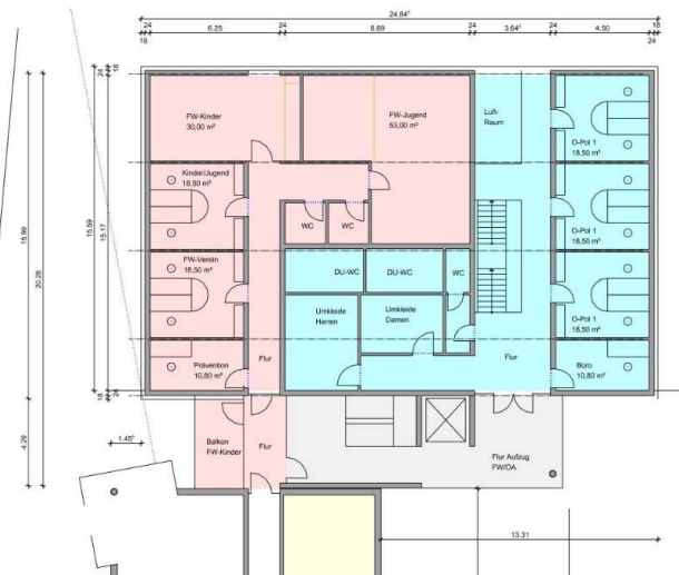
1. OG – Verwaltungsbau
