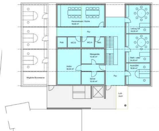
2. OG – Verwaltungsbau
