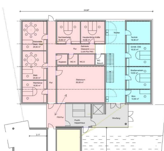
EG – Verwaltungsbau
