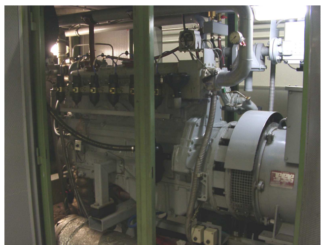
[Bild 19 + 20: links → Gasbehälter; rechts → Blockheizkraftwerk (BHKW)]
