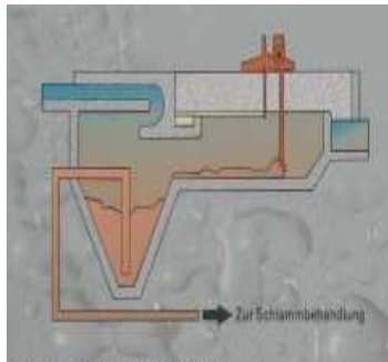
[Graphik 7: Vorklärung]
