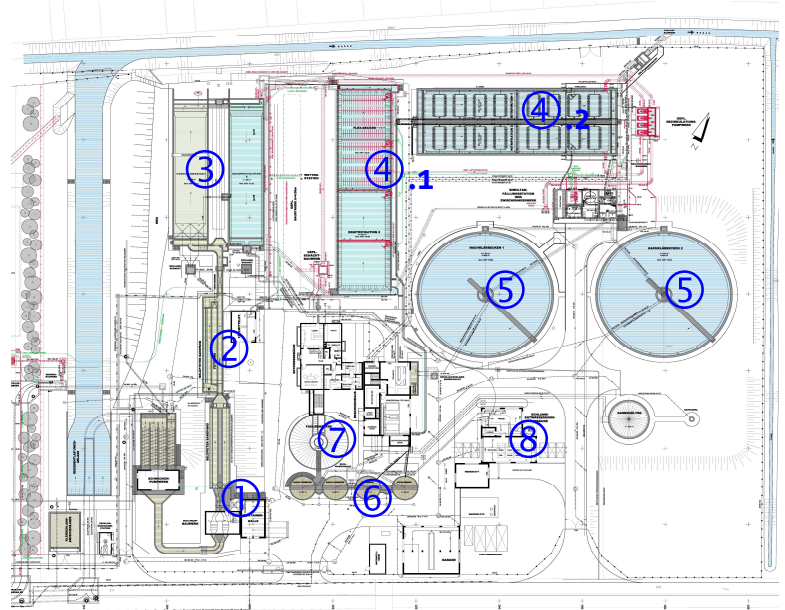
[Graphik 4: Fliesbild der Kläranlage Ober-Roden]
