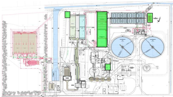
[Graphik 13: Kläranlage Ober-Roden 2008, Umbau bzw. Umbau gem. obiger Auflistung (grün hervorgehoben)]
