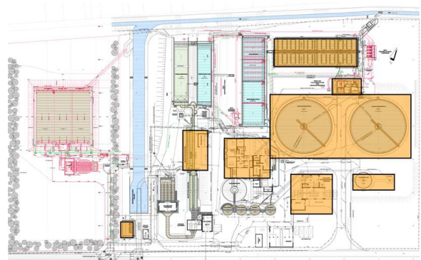
[Graphik 12: Kläranlage Ober-Roden 1999, neue Anlageteile bestehend aus Fäkalannahmestation, Sand-/ Fettfang, Belüftung, Nitrifikation, Nachklärbecken, Schlammwässerung, Gasbehälter (orange hervorgehoben)]
