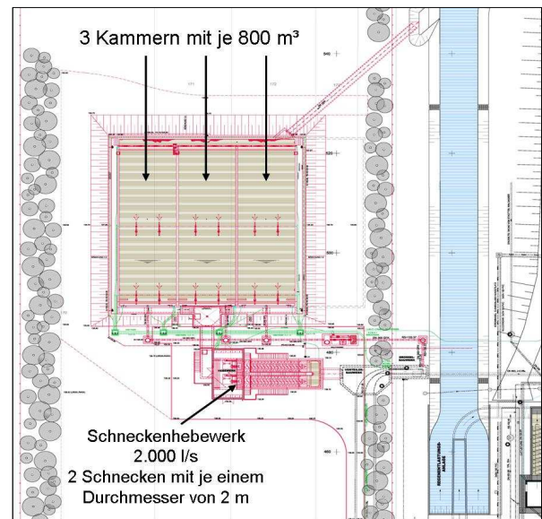
[Graphik 14: Frachtspeicher- u. Pufferbecken]
